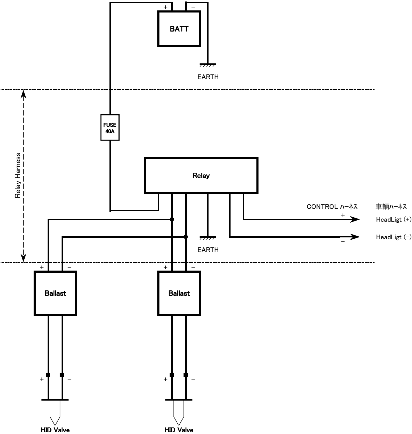
Wagon R RR (MC21) HID 取付配線図
